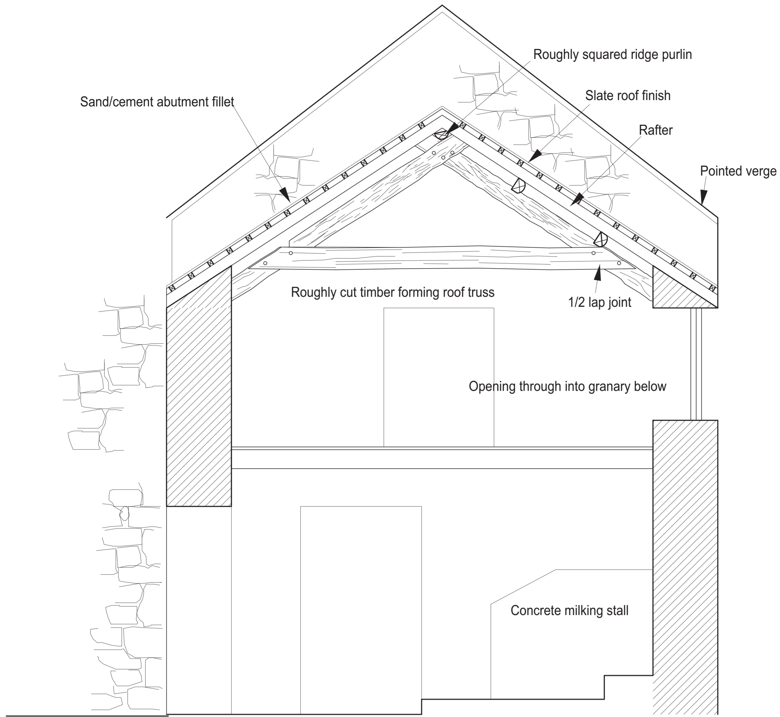
Section a-a
