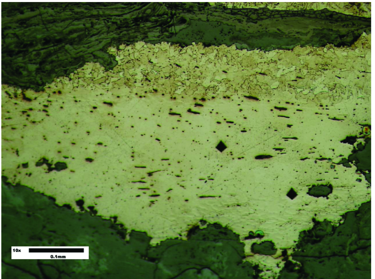
Plate 7.3.1 Composite bars
