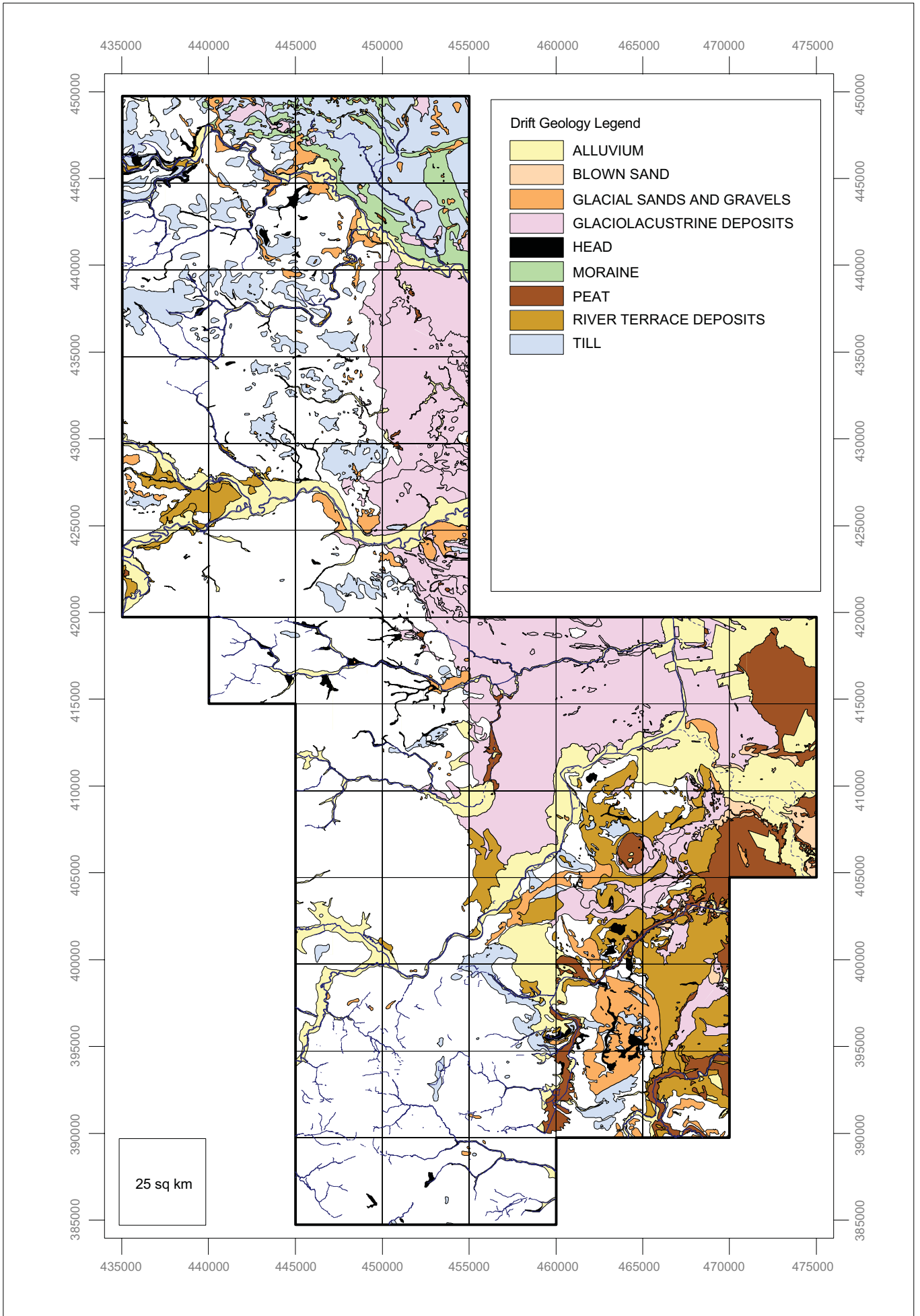
Fig. 1.3. Drift geology
