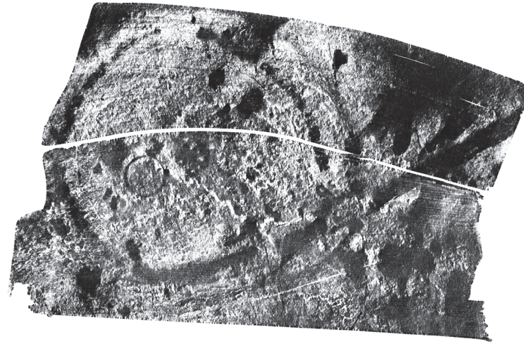
55.0 - 57.5ns (2.64 - 2.76m)
