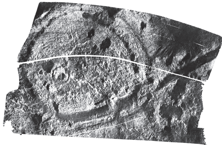
37.5 - 40.0ns (1.45 - 1.55m)
