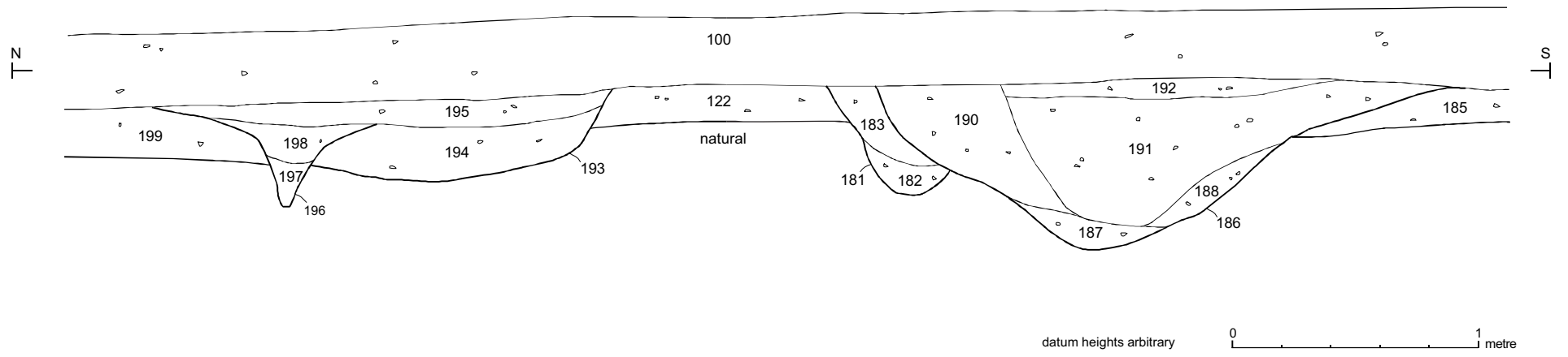
Fig. 7 Section 10. Scale 1:25.
