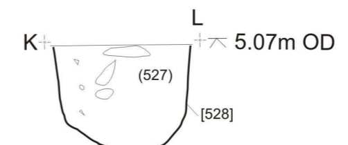
Fig. G. West Section
