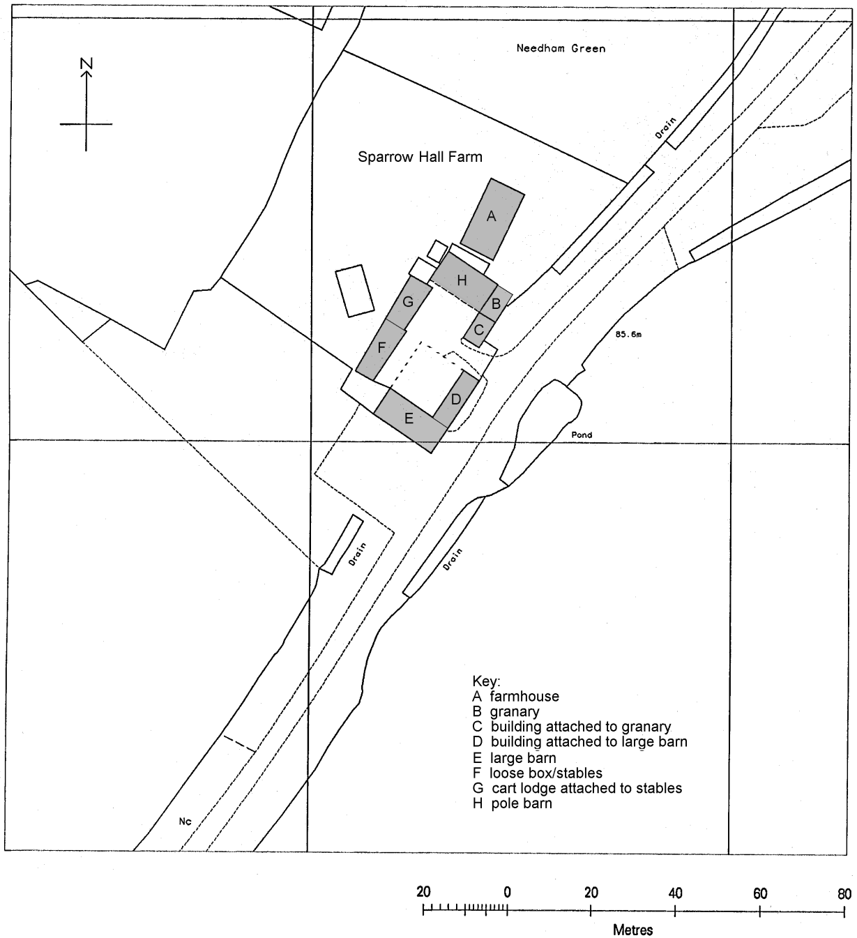
Fig 6 Site plan.
