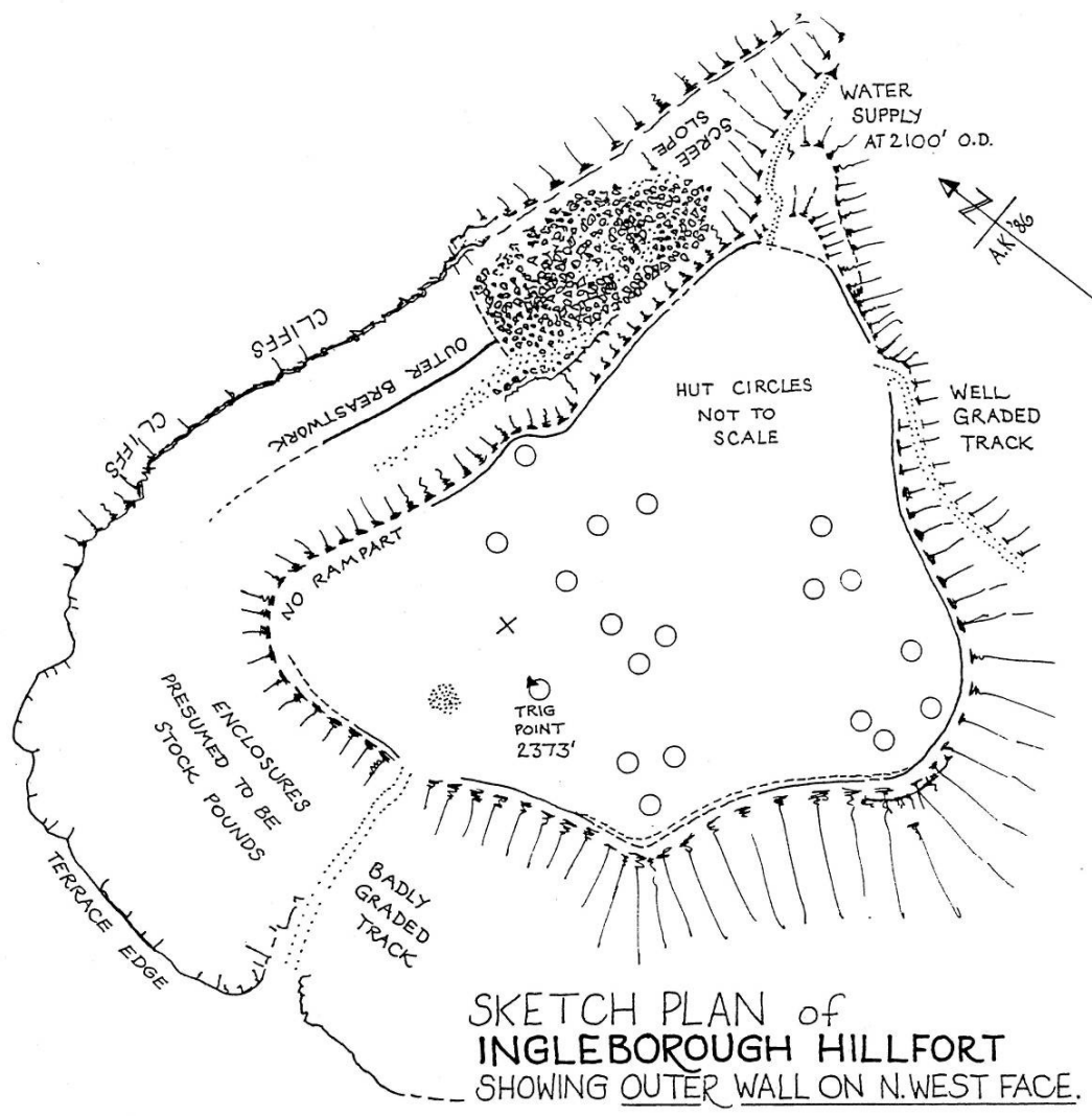
FIG. 1. SITE PLAN
